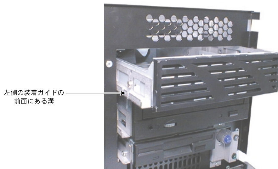
図9-5 デバイストレイの挿入
