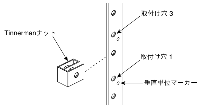
図 1-1 Tinnerman ナットの取付け穴への取り付け
