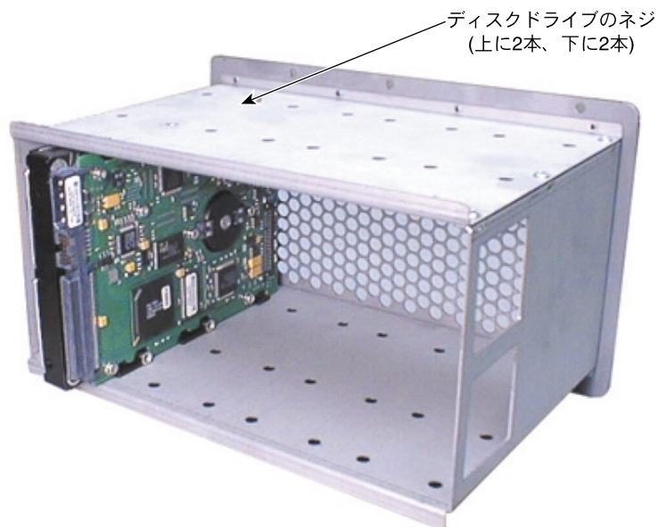
図9-7 ディスクドライブケージ
