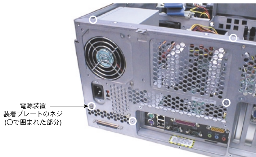
図9-11 電源装置の装着ネジ
