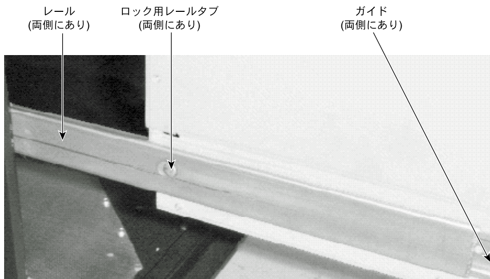
図1-8 レールガイドとレール
