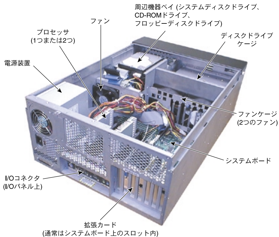
図 7-2 内部のシステムコンポーネント
