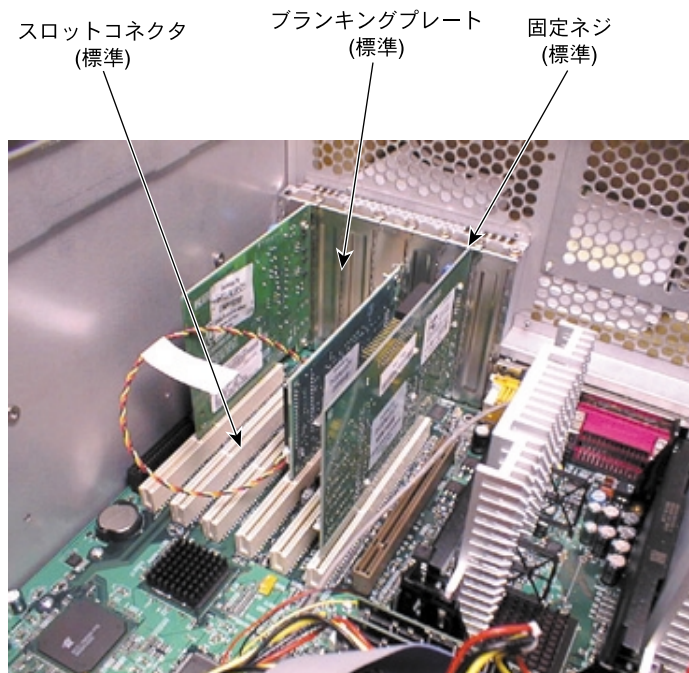
図8-2 拡張カード
