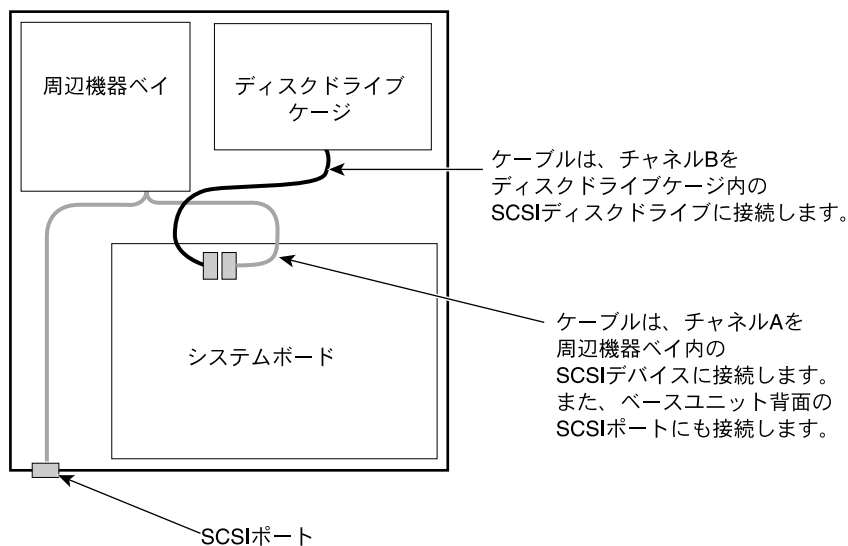
図 10-3 SCSIケーブル
