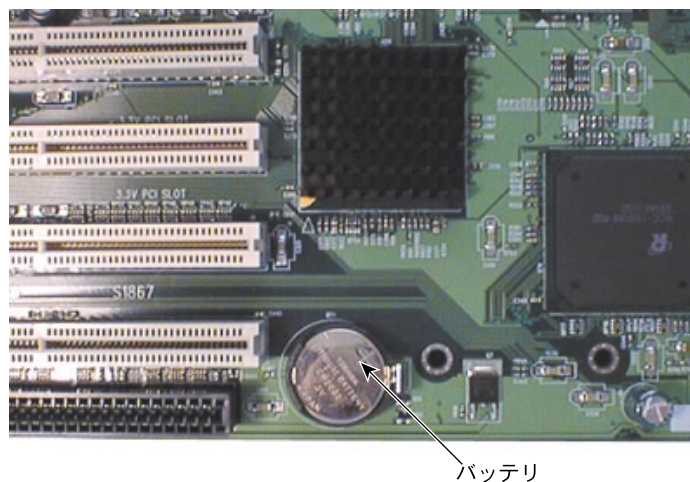
図9-18 CMOS/クロックリチウムバッテリー
