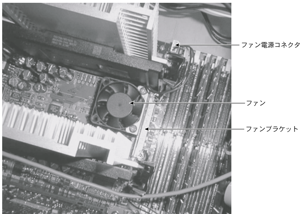
図9-16 プロセッサ領域の冷却ファン
