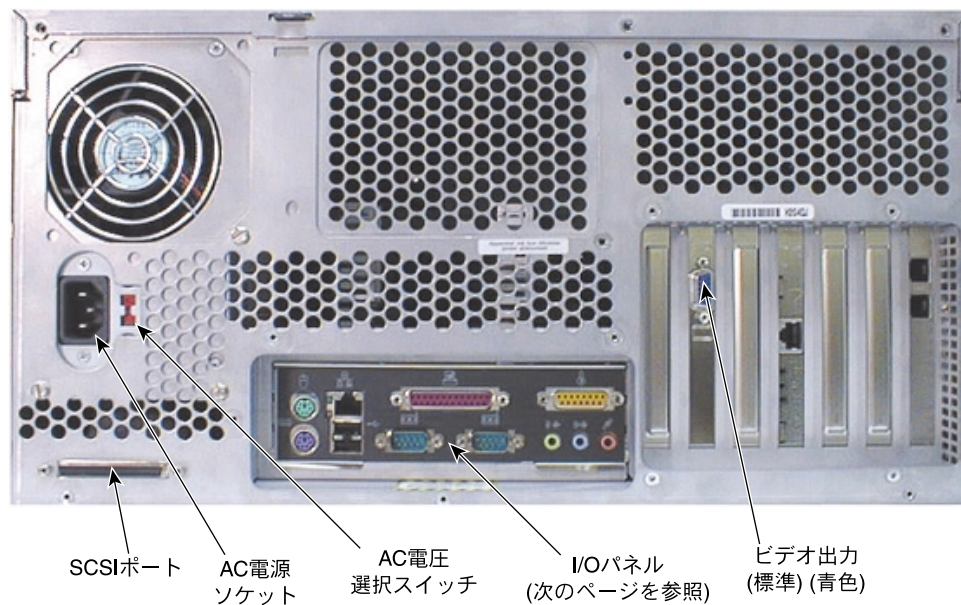
図1-9 ベースユニットの背面
