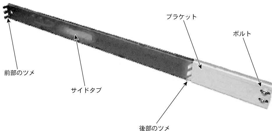
図1-4 レールブラケットの部品
