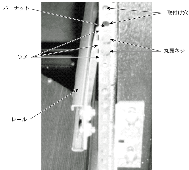
図1-5 ラックの前面マウントレールに取り付けたレール
