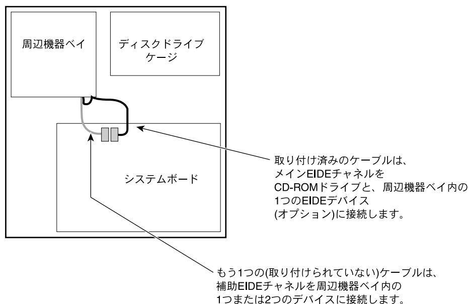
図 10-2 EIDE ケーブル
