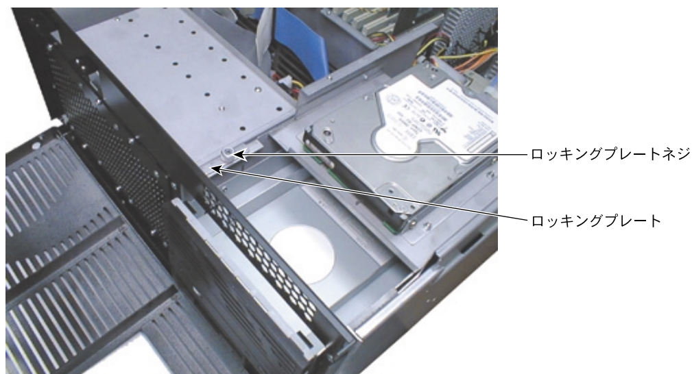
図9-3 デバイストレイのロックングプレート
