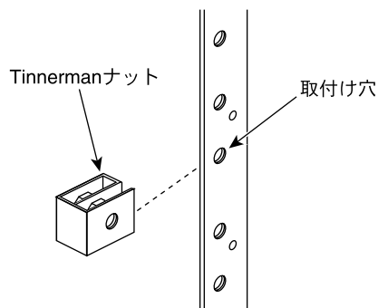
図 1-6 Tinnerman ナットの取付け穴への取り付け
