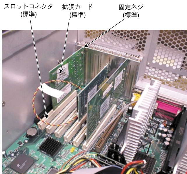
図9-8 搭載されている拡張カード
