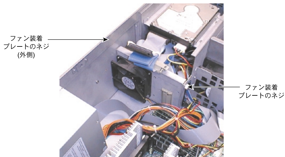
図9-14 リアファン
