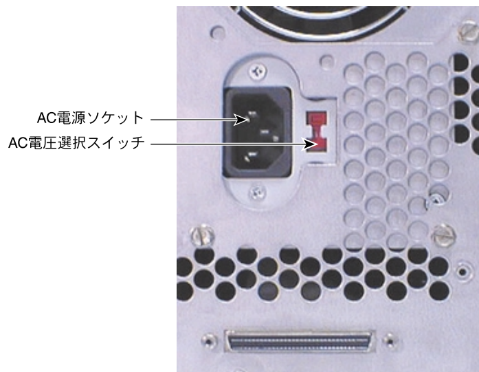
図 1-12 AC 電源
