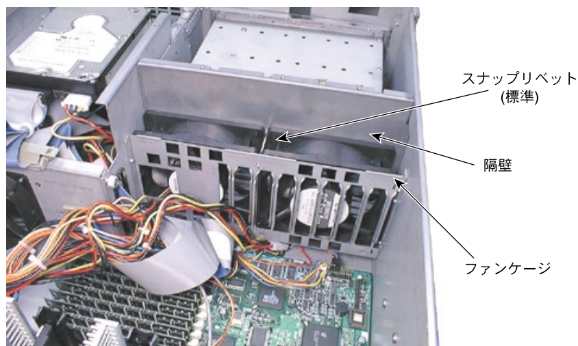
図9-15 フロントファン
