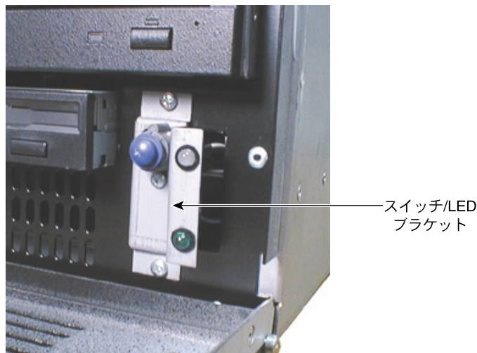
図9-19 電源スイッチ /LED ブラケット
