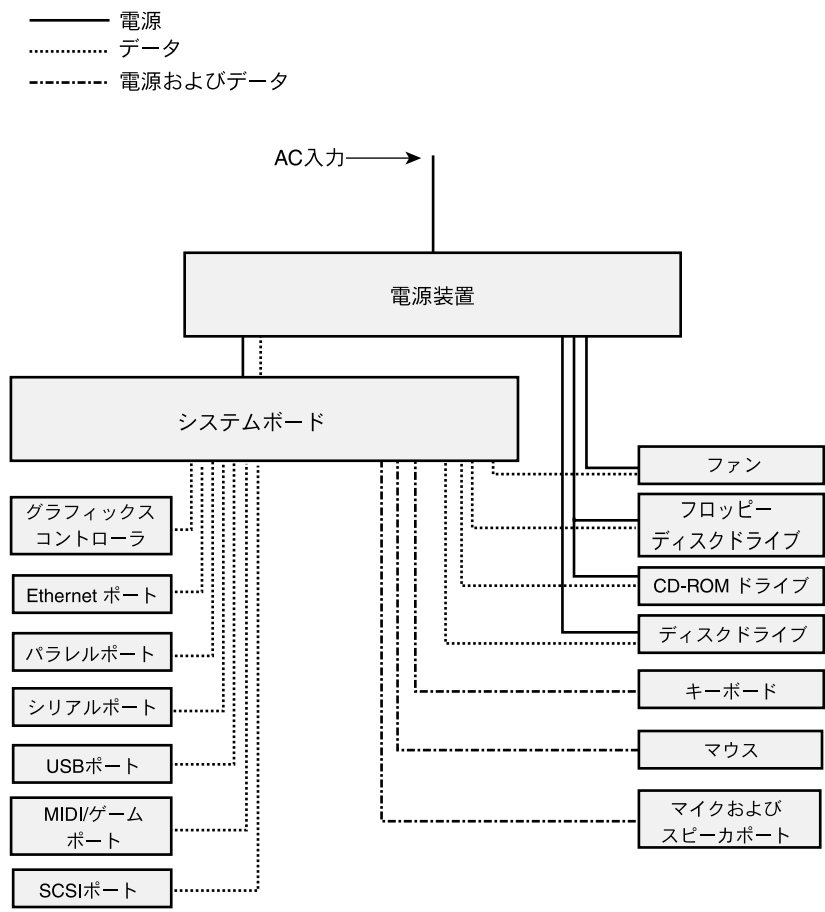
図 10-1 電源およびデータ信号の図
