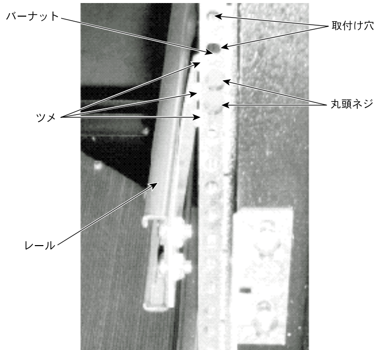
図1-7 ラックの背面マウントレールに取り付けたレール
