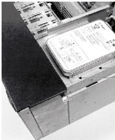
図9-2 システムディスクドライブ
