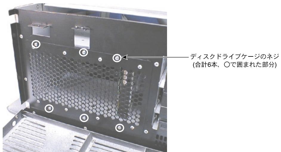
図9-6 搭載されているディスクドライブケース
