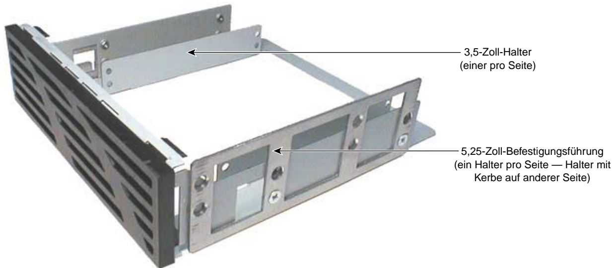
Abbildung 9-4 Geräteträger
