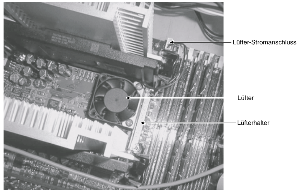
Abbildung 9-16 Prozessorbereichslüfter
