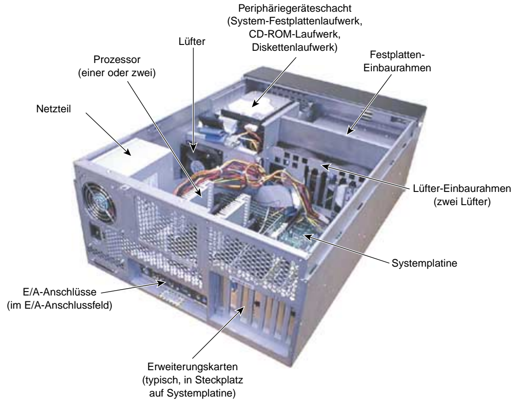
Abbildung 7-2 Interne Systemkomponenten
