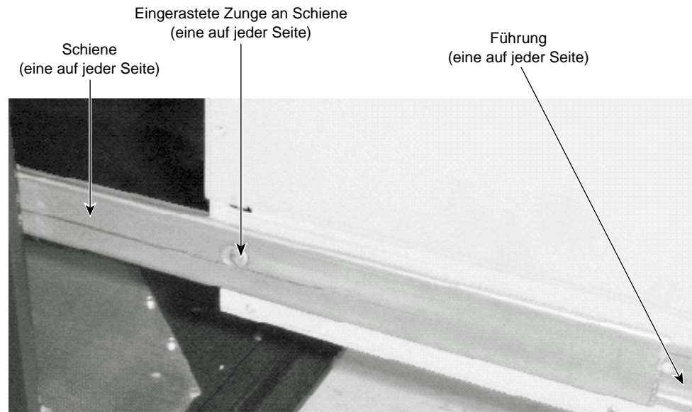
Abbildung 1-8 Schiene und Führungsleiste
