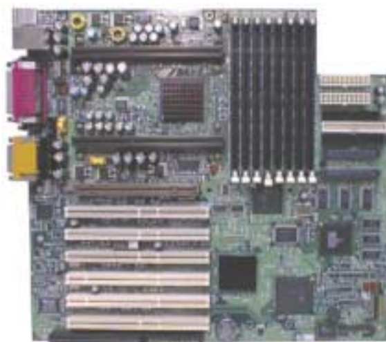
Abbildung 9-17 Die Systemplatine
