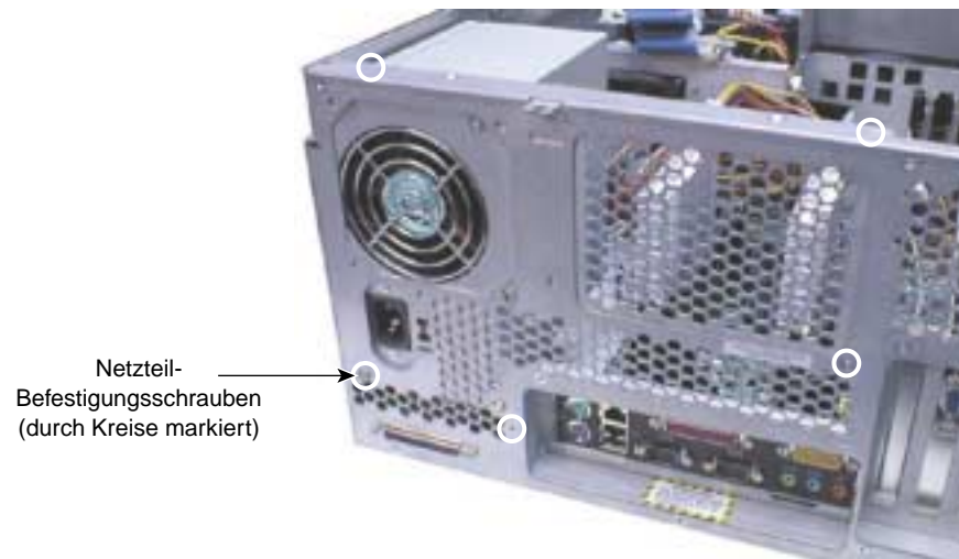
Abbildung 9-11 Befestigungsschrauben für das Netzteil
