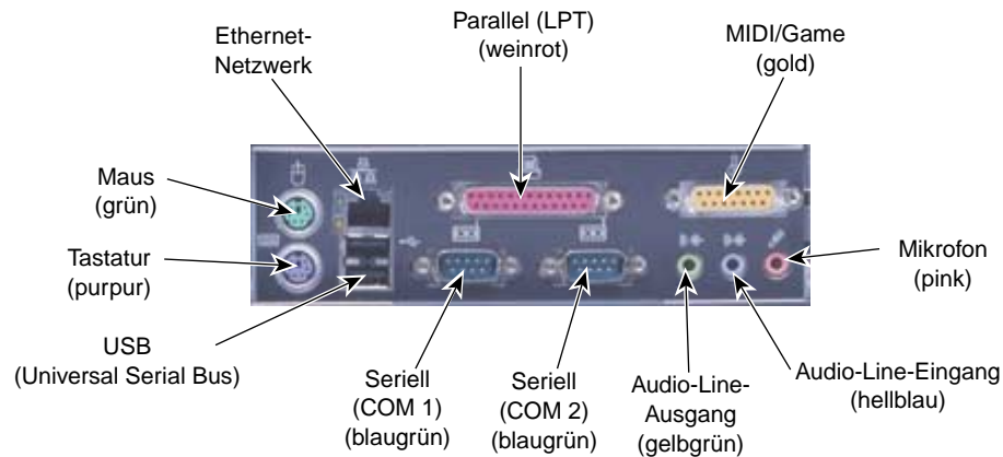
Abbildung 1-10 E/A-Anschlussfeld (Eingänge und Ausgänge)
