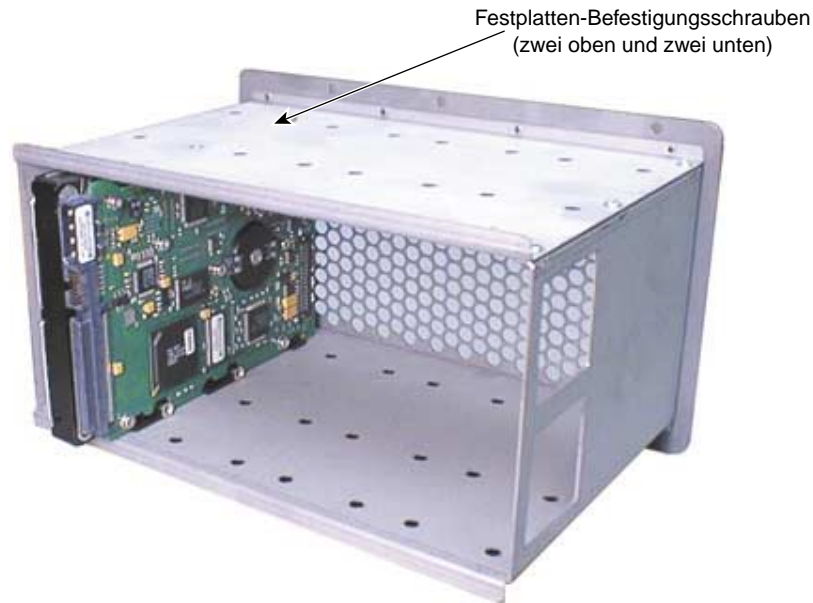
Abbildung 9-7 Festplatten-Einbaurahmen
