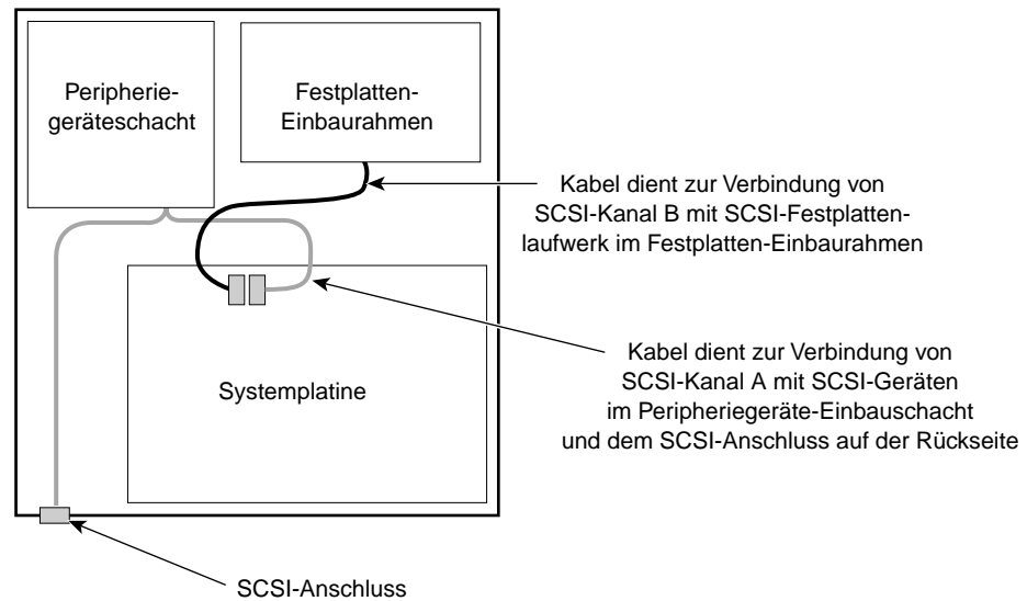
Abbildung 10-3 SCSI-Kabel
