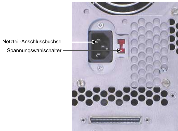
Abbildung 1-12 Stromversorgung
