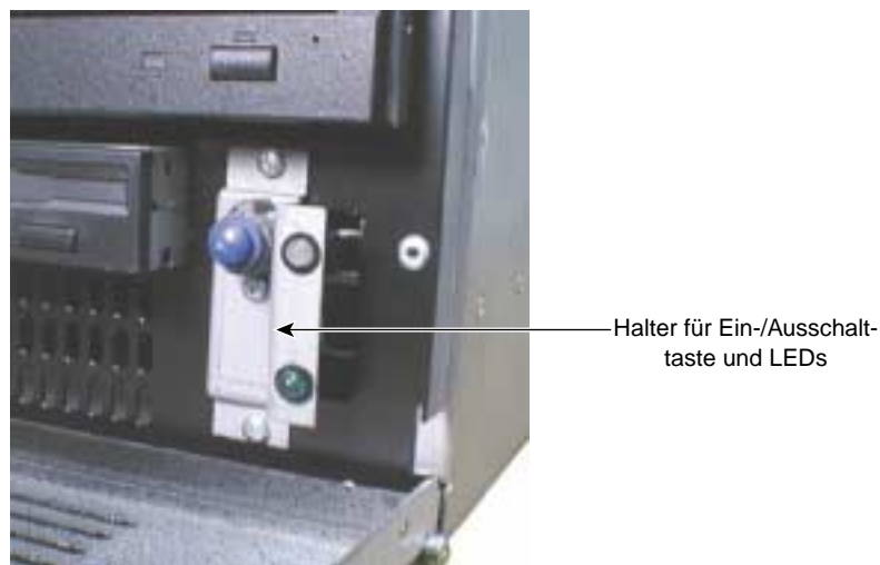
Abbildung 9-19 Ein-/Ausschalttaste und LED-Halter
