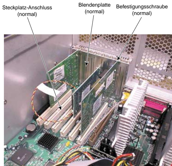
Abbildung 8-2 Erweiterungskarten
