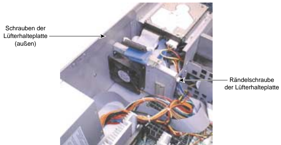
Abbildung 9-14 Hinterer Lüfter
