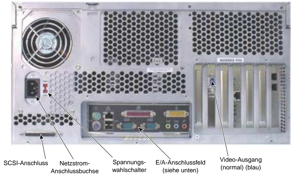
Abbildung 1-9 Rückseite des Rechners
