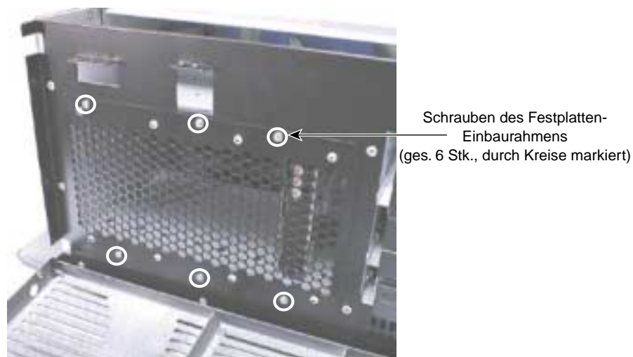
Abbildung 9-6 Festplatten-Einbaurahmen eingebaut
