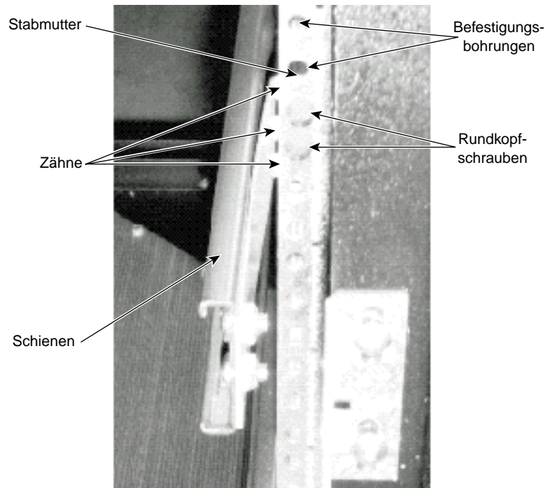
Abbildung 1-7 Befestigung einer Schiene an der hinteren Montageschiene des Geräte-Racks
