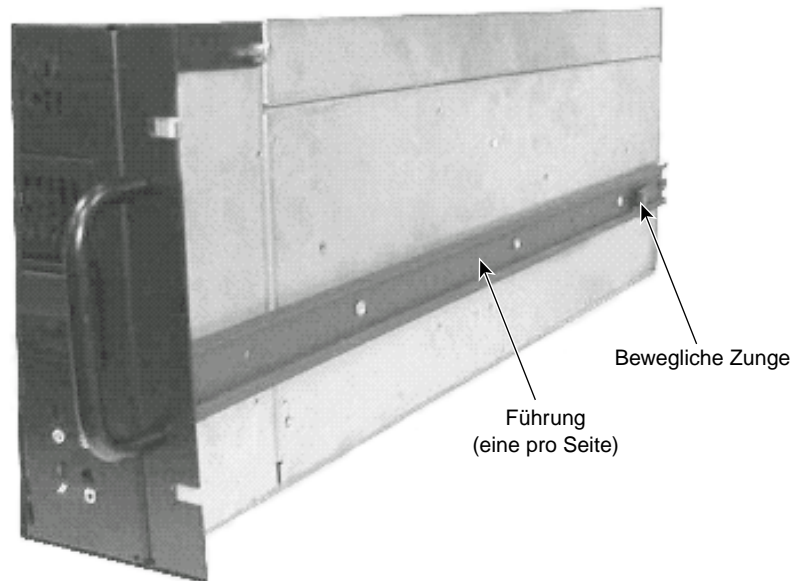
Abbildung 1-3 Die Führungsleiste
