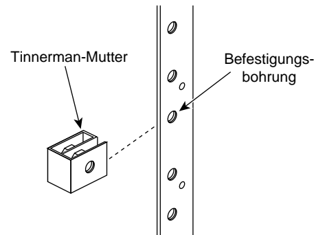
Abbildung 1-6 Anbringen einer Tinnerman-Mutter an einer Befestigungsbohrung
