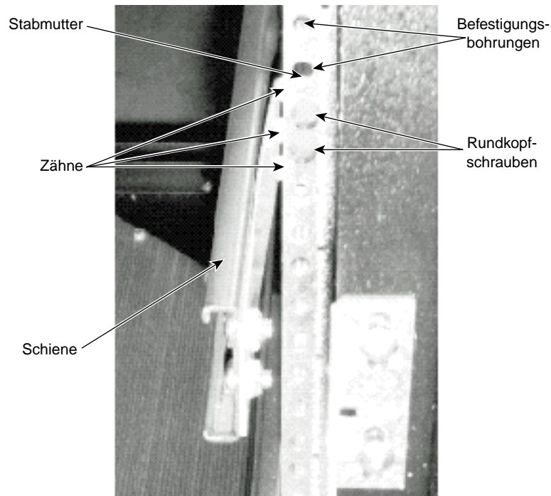
Abbildung 1-5 Befestigung eine Schiene an der vorderen Montageschiene des Geräte-Racks
