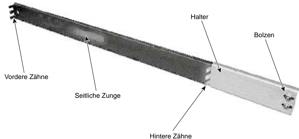
Abbildung 1-4 Teile der Schienenhalterung
