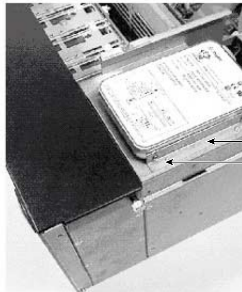
Abbildung 9-2 System-Festplattenlaufwerk
