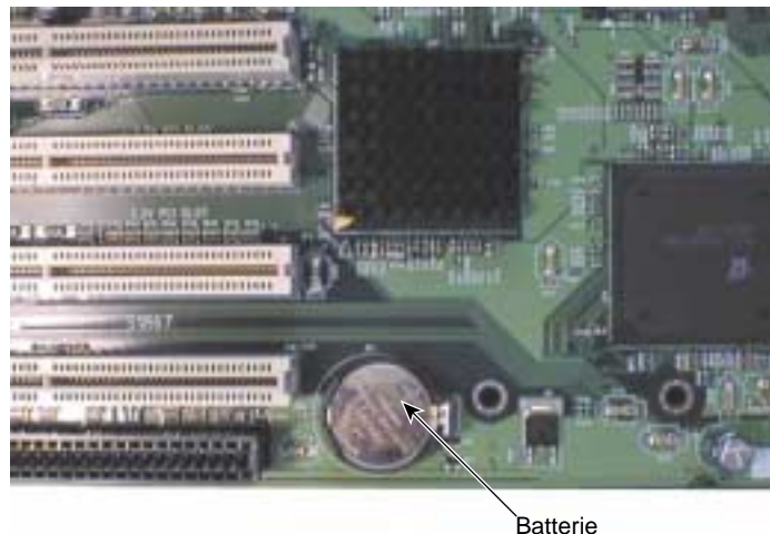
Abbildung 9-18 Lithiumbatterie von CMOS und Systemuhr
