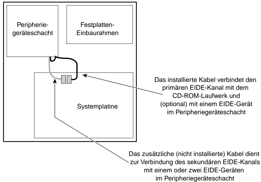
Abbildung 10-2 EIDE-Kabel
