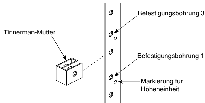
Abbildung 1-1 Montage einer Tinnerman-Mutter an einer Befestigungsbohrung
