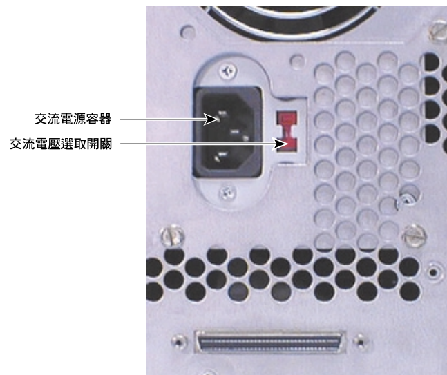
圖9-13 交流電
