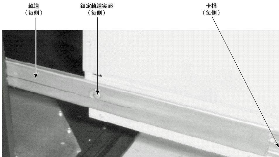
圖 1-8 軌道卡榫上的軌道
