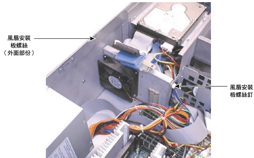
圖9-14 後風扇
