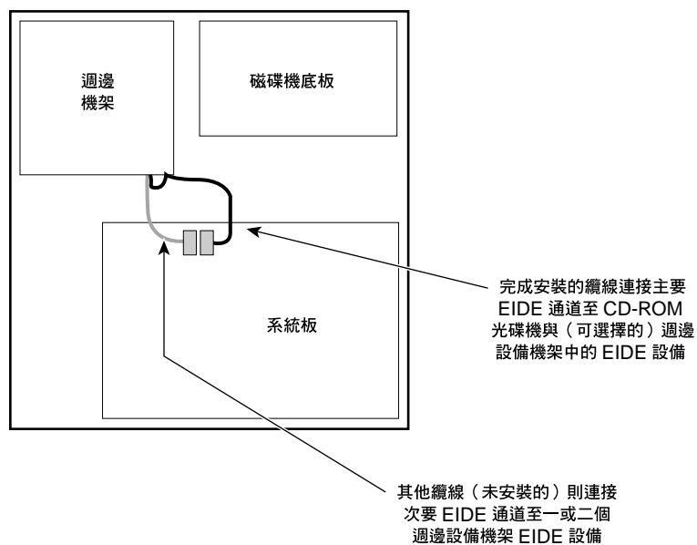
圖 10-2 EIDE 電纜
