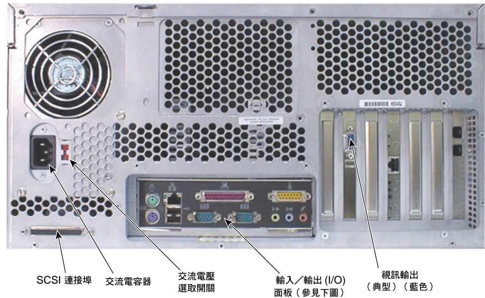
圖 1-9 基本單元背面
