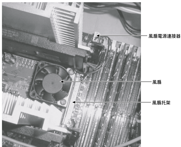
圖 9-16 處理器區冷卻風扇
