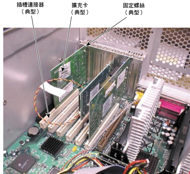
圖 9-8 完成安裝的擴充卡
