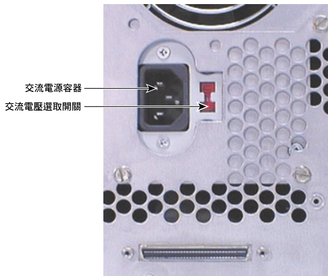
圖 1-12 交流電
