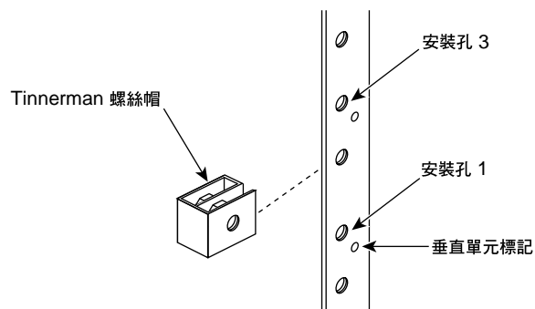
圖 1-1 在安裝孔中安裝 Tinnerman 螺絲帽
