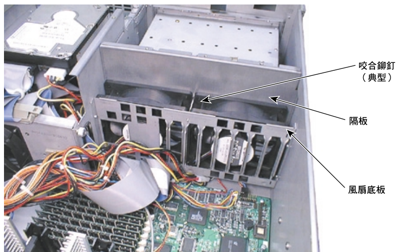
圖9-15 前風扇
