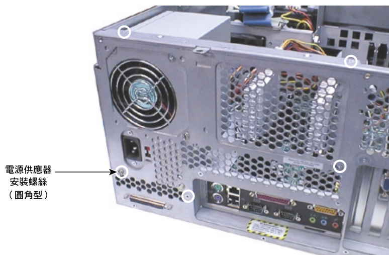
圖9-11 電源供應器安裝螺絲
