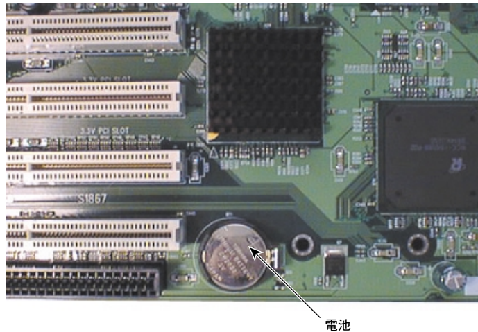
圖 9-18 CMOS/Clock 鋰電池
