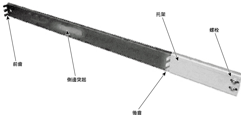
圖 1-4 軌道托架零件
