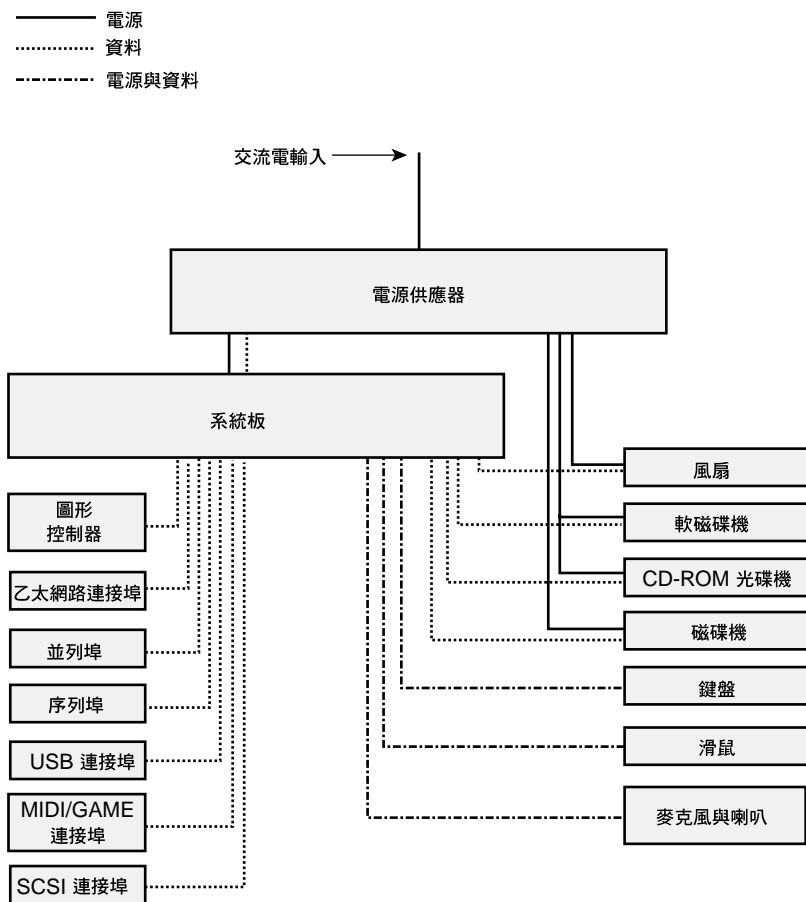
圖 10-1 電源和資料信號圖解
