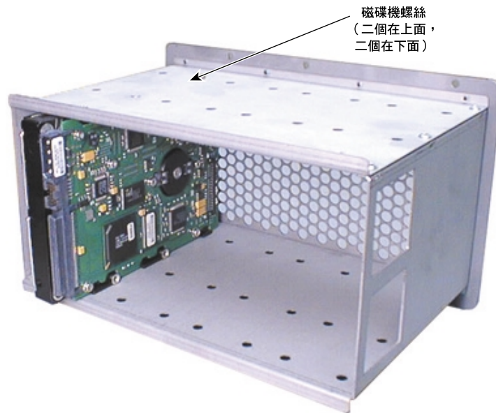
圖 9-7 磁碟機底板
