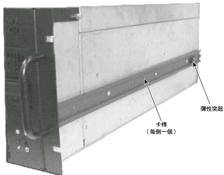
圖 1-3 軌道卡榫
