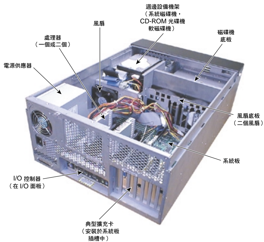
圖 7-2 內部系統組件
