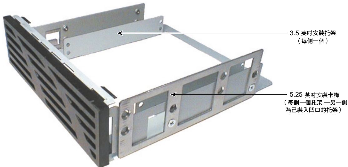
圖 9-4 設備托盤
