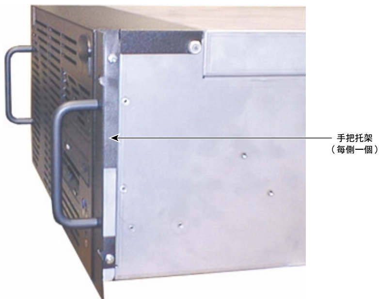
圖 1-2 基本單元手把托架
