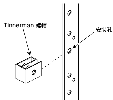
圖 1-6 安裝 Tinnerman 螺帽到一個安裝孔中
