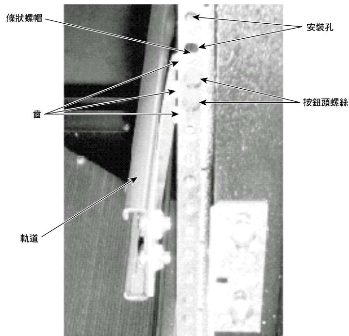
圖 1-5 安裝設備框架的前安裝軌道上的軌道
