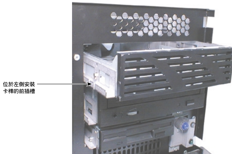
圖 9-5 插入設備托盤
