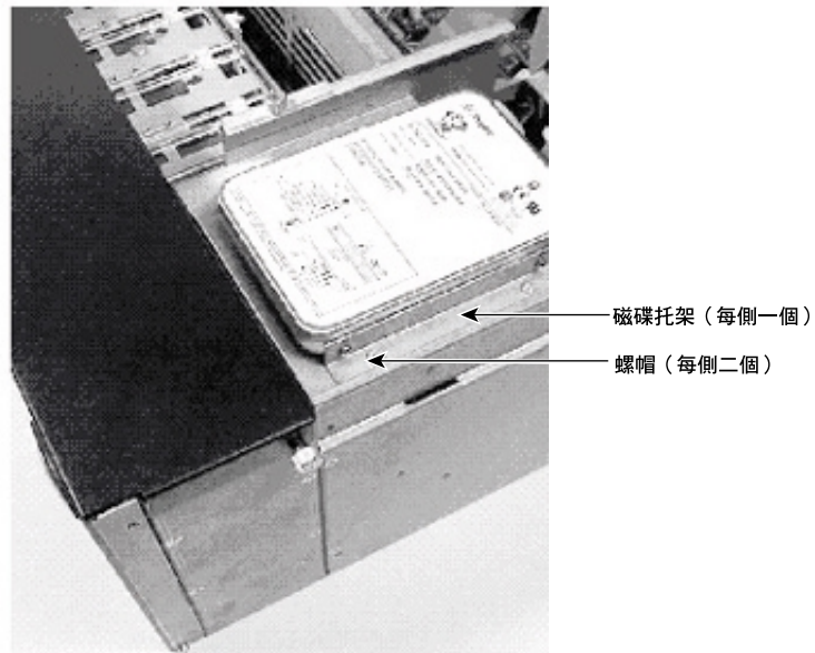
圖 9-2 系統磁碟機
