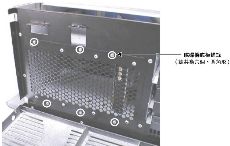
圖 9-6 完成安裝的磁碟機底板
