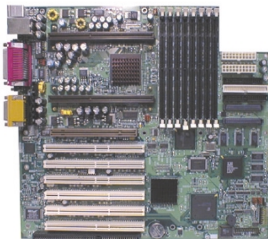
圖 9-17 系統板
