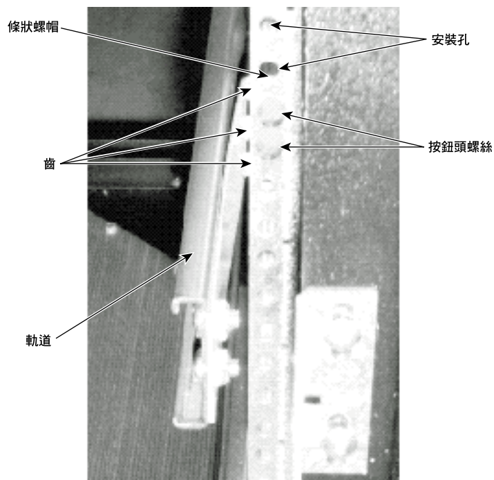
圖 1-7 安裝設備框架的前安裝軌道上的軌道
