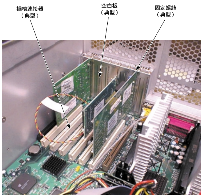
圖 8-2 擴充卡
