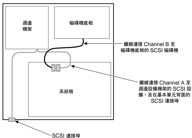
圖 10-3 SCSI 電纜
