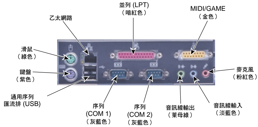
圖 1-10 輸入／輸出 (I/O) 面板
