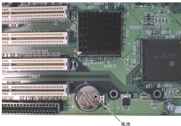
图 9-18 CMOS / 时钟锂电池
