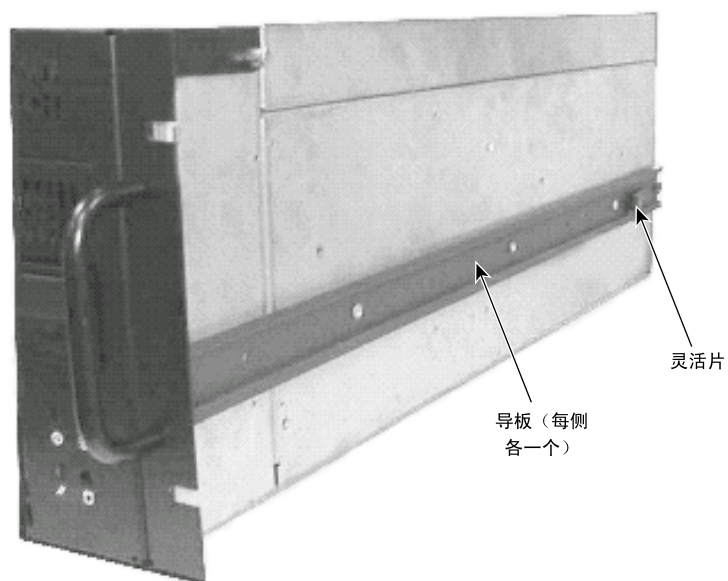
图 1-3 滑导轨板
