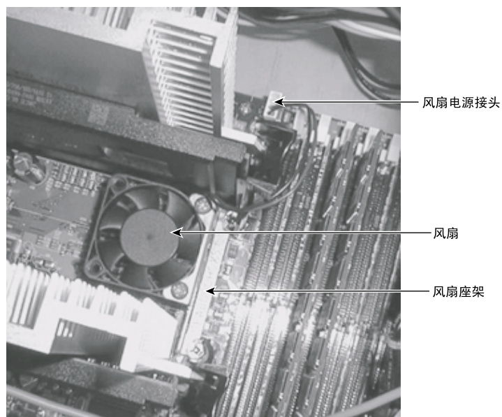
图 9-16 处理器区域的冷却风扇
