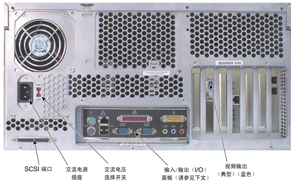
图 1-9 主机箱的背面
