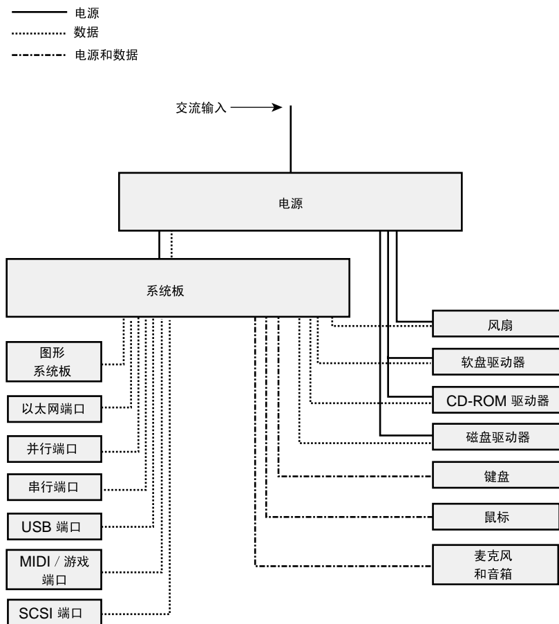
图 10-1 电源和数据信号图表
