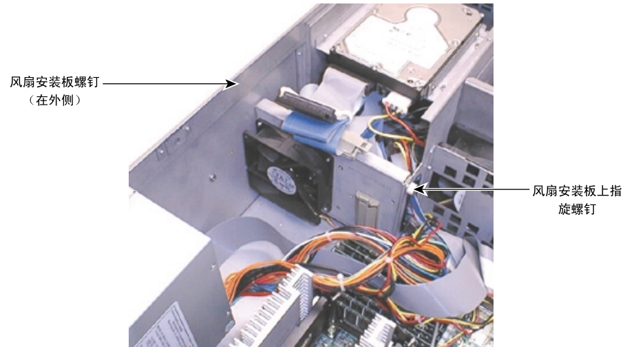
图 9-14 后置风扇
