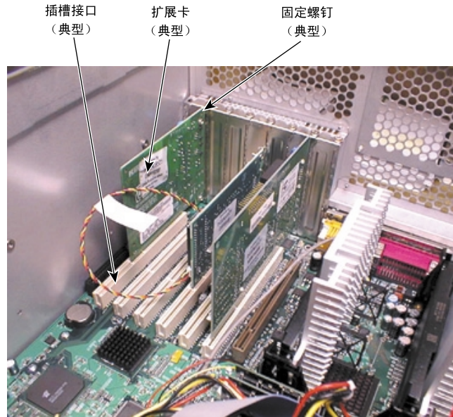
图 9-8 安装扩展卡
