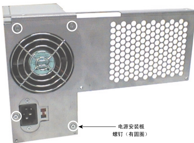
图9-12 电源安装板
