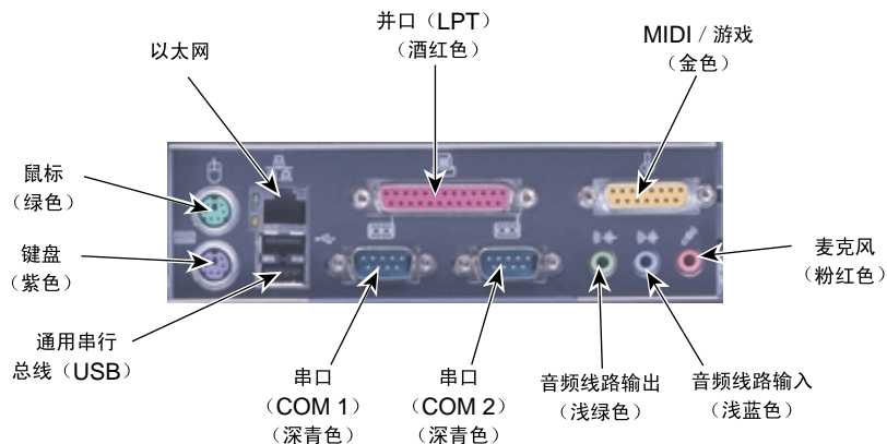
图 1-10 输入 / 输出 (I/O) 面板
