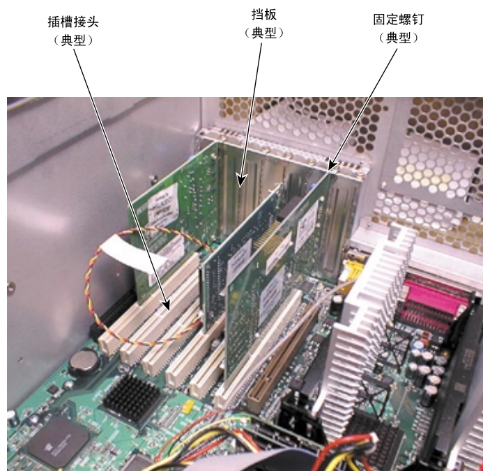
图 8-2 扩展卡
