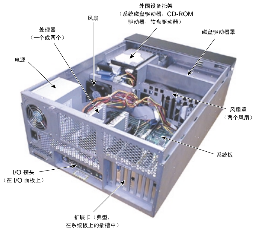
图 7-2 内部系统部件
