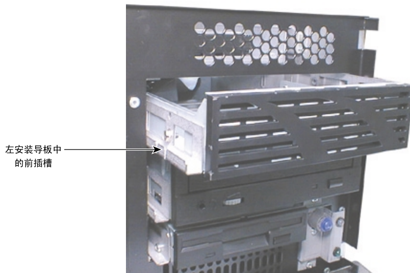
图 9-5 插入设备支架
