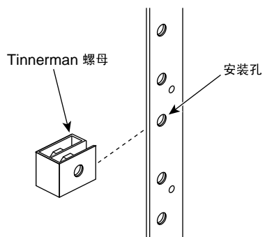
图 1-6 将Tinnerman 螺母安装到安装孔中
