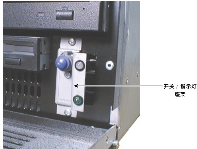
图9-19 电源开关 / 指示灯座架
