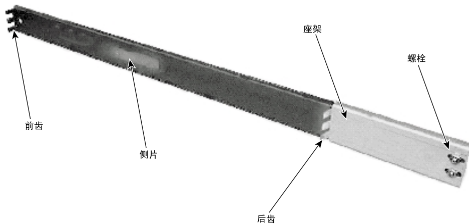
图 1-4 滑轨座架部件
