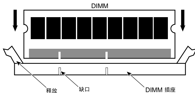
图 9-9 双列直插式内存条 (DIMM)
