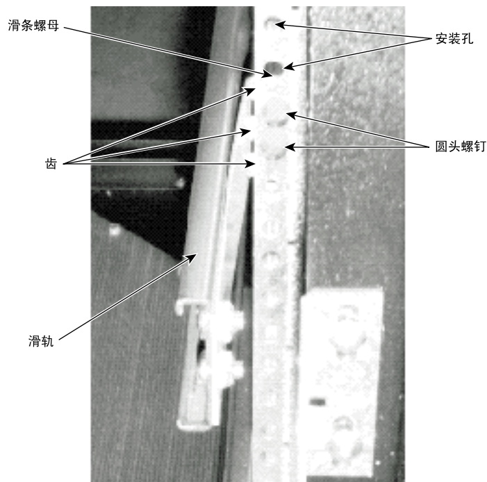
图 1-7 固定到机架的后安装滑轨的滑轨
