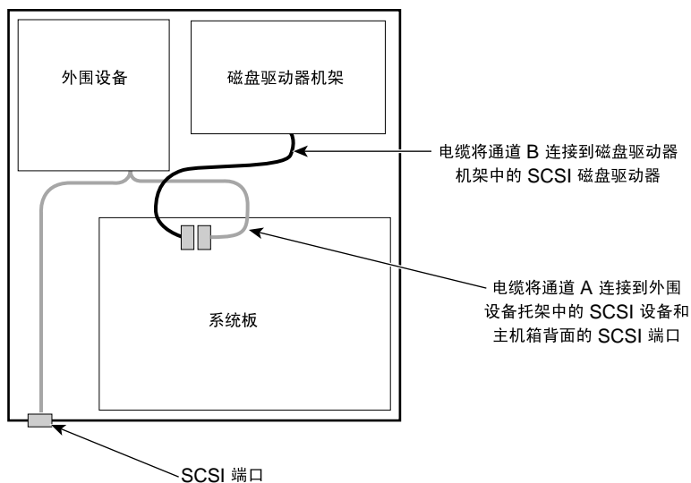
图 10-3 SCSI 电缆
