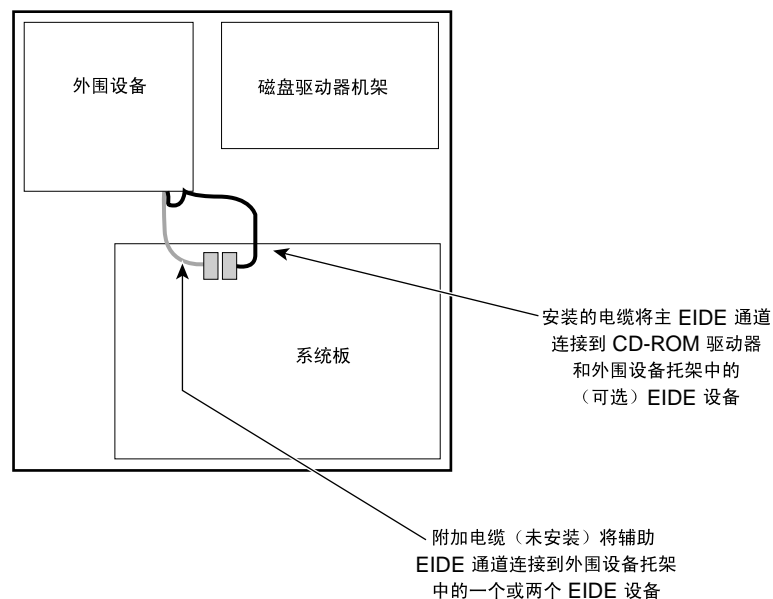
图 10-2 EIDE 电缆
