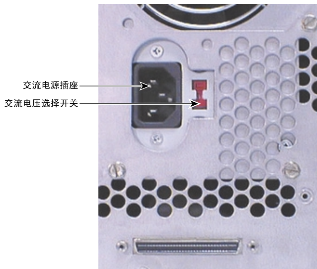
图 1-12 交流电源
