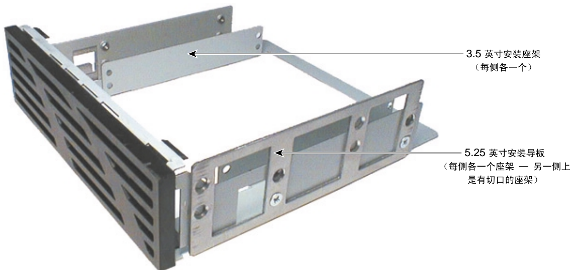
图 9-4 设备支架
