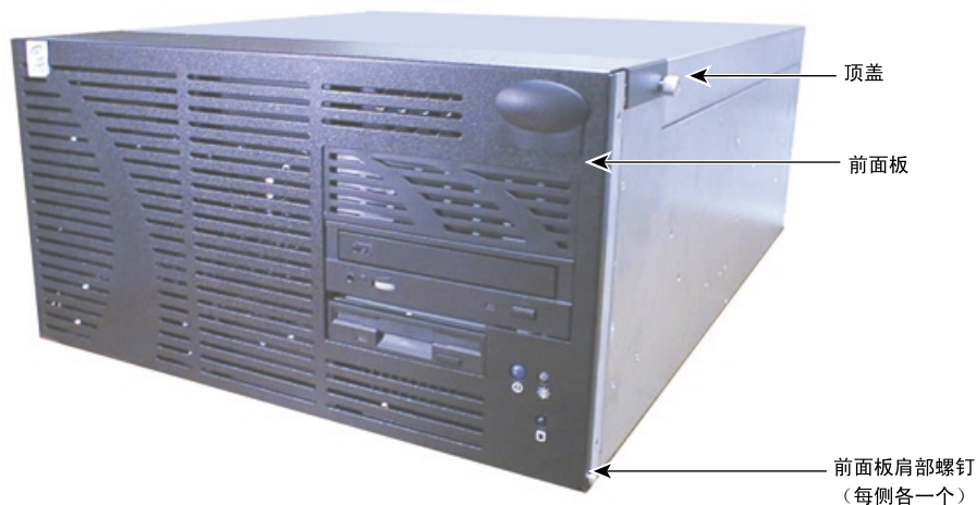
图9-1 主机箱的机箱部件
