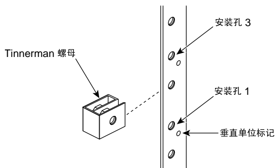
图 1-1 将 Tinnerman 螺母安装到安装孔中
