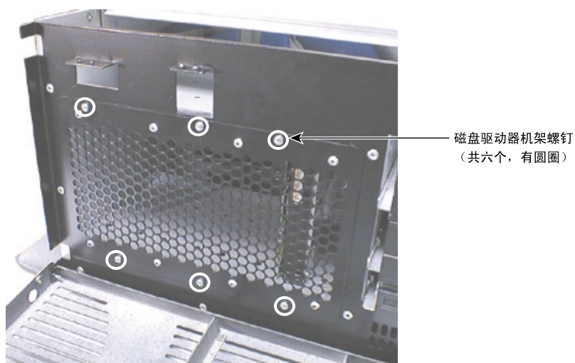
图9-6 安装的磁盘驱动器仓
