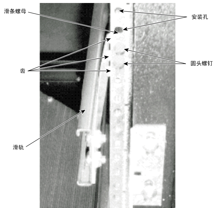
图 1-5 固定到机架前安装滑轨的滑轨
