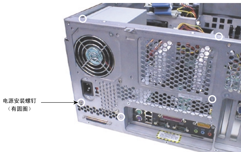
图9-11 电源安装螺钉
